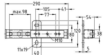
Glissière coulissante M10
